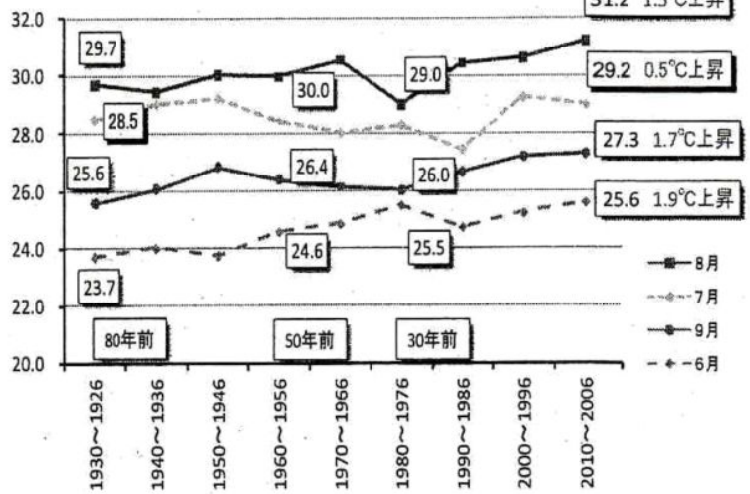
日最高気温の月平均(5年平均、横浜)
